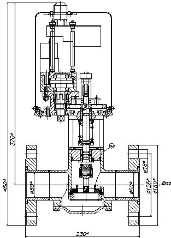
Рис.1 Габаритные размеры клапана
